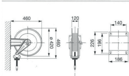
Dimensioner - ydermål (mm) Serie 430 åben ABS fast
