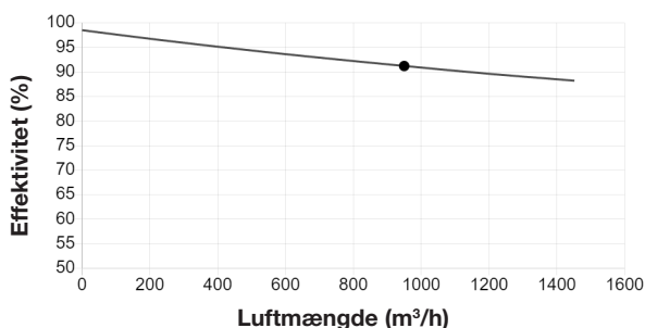
Temperaturvirkningsgrad
