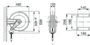
Dimensioner - ydermål (mm) Serie 430 åben ABS fast
